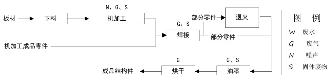
图 3-5 组件机加工工艺流程及排污节点
